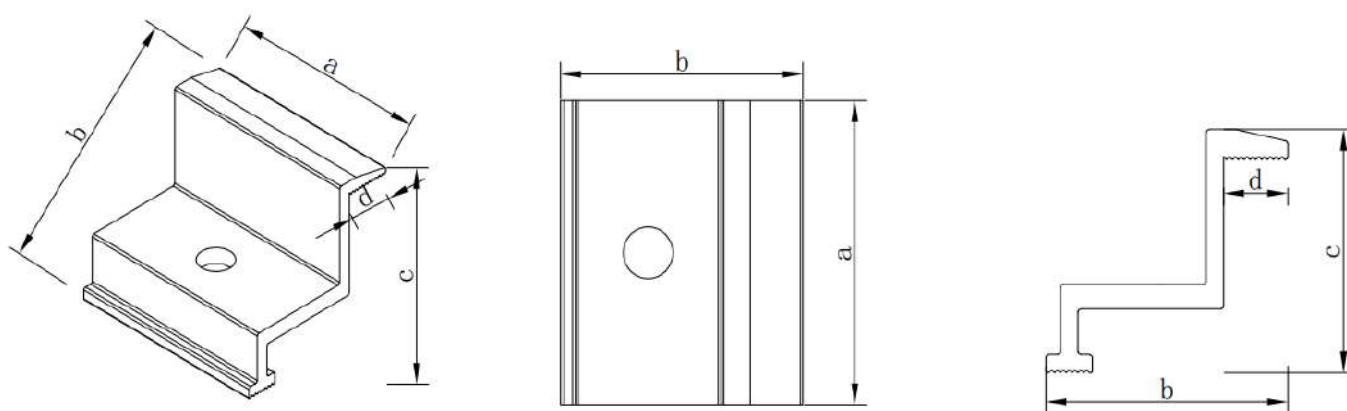
Fig. 5 Clamp
